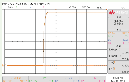
HY-HV 10kV-50mA满载上升时间:101ms
