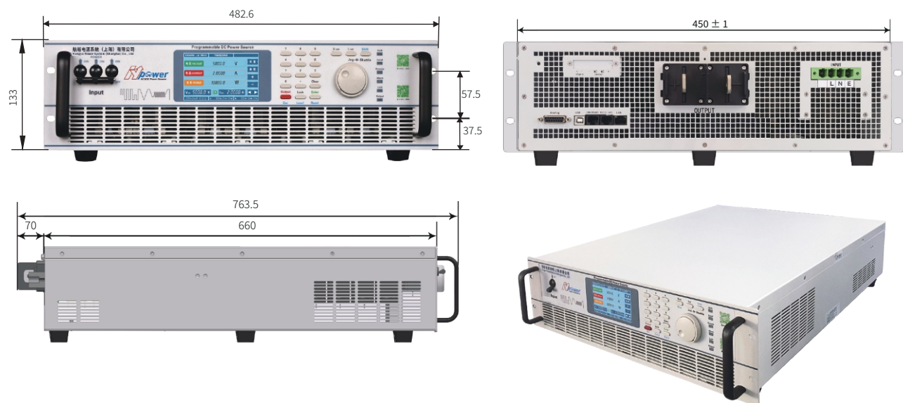
3U 机型 450(W) * 660(D) * 133(H) mm
