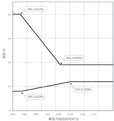
GJB 181B-2012 图12 28V直流正常瞬变电压包络线
