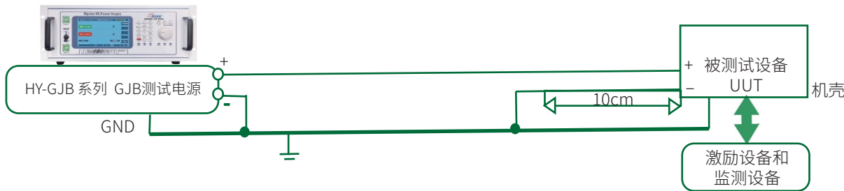
图HDC302-1 非正常电压瞬变试验系统典型配置
