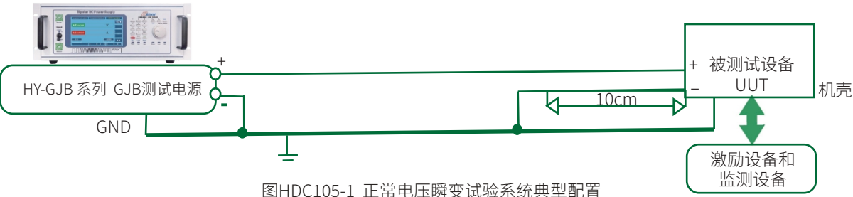
图HDC105-1 正常电压瞬变试验系统典型配置
